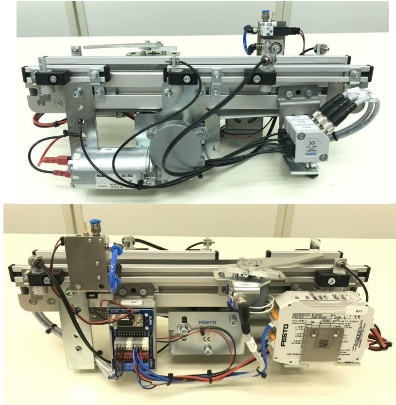
図4 コンベアモジュールの持ち込み状態
