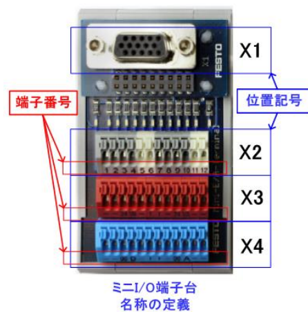
図5 ミニ I/O 端子台
